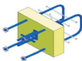
Avec barres de raccordement et ancrages terminaux raccourcis (console en 2 ème étape).
