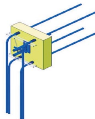
Avec prolongement d'étrier de traction en 1 ère étape.
