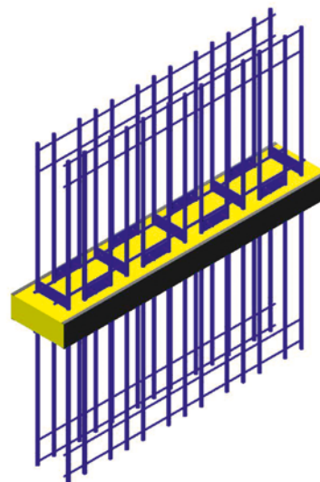
Éléments en M avec rigidification en H bidirectionnelle – et beaucoup d'autres options de conception. Nos ingénieurs se font un plaisir de vous conseiller.
