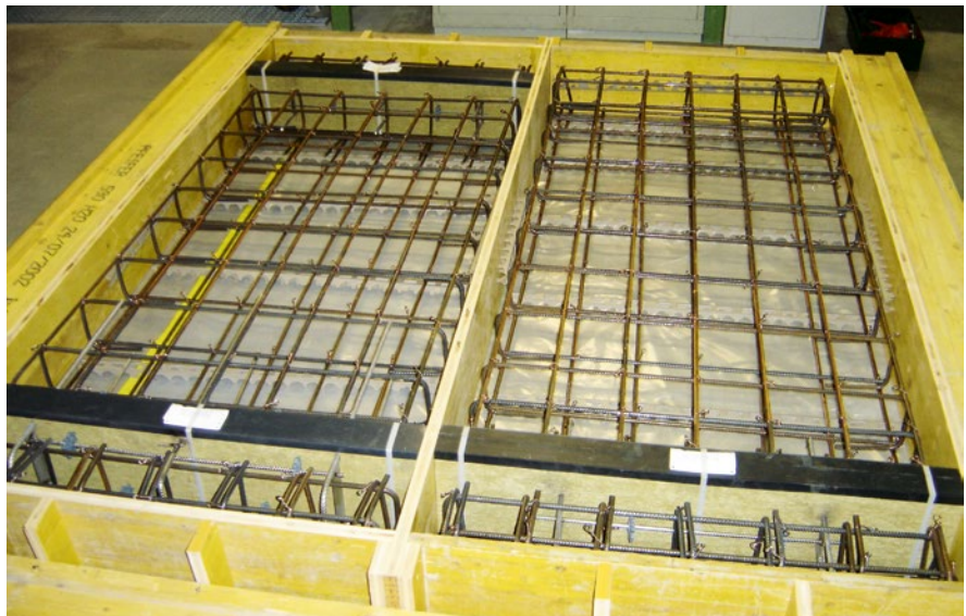
Armature des dalles d'essais. A gauche : avec Ancon-Iso, à droite: dalle de référence intégrale en béton.
