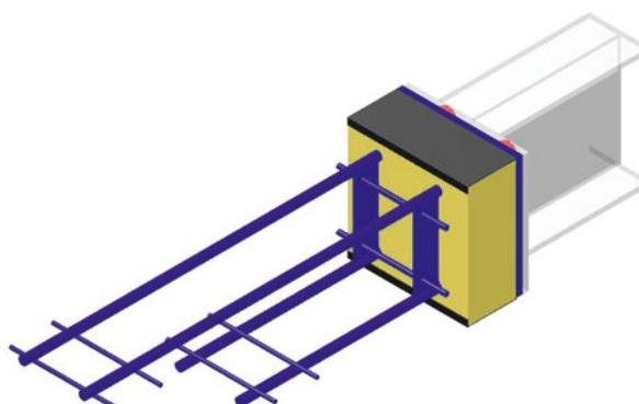
Connecteur en acier pour profil porteur
