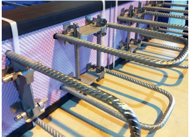
Éléments pour embases de murs spéciaux
