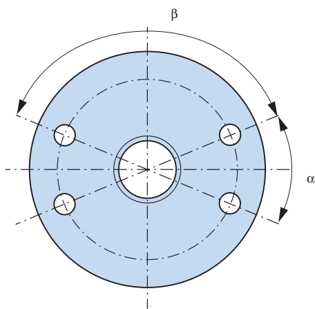
1. Exemple de référence de commande : Disque de répartition, Detan-S, d_s = 42 mm, 4 trous \alpha = 40^\circ , \beta = 140^\circ (voir dessin), FV
