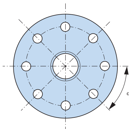
2. Exemple de commande (matériau : acier inoxydable) : Disque de répartition, Detan-D, d_s = 24 mm, 8 trous \alpha = 45^\circ (voir dessin)
