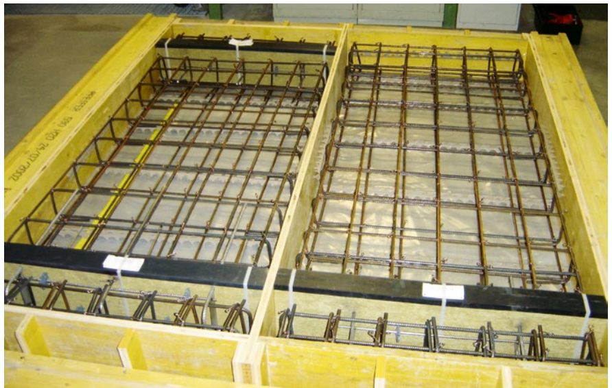
Bewehrung der Versuchsplatten. Links: mit Ancon-Iso, rechts: Referenzplatte durchbetoniert.
