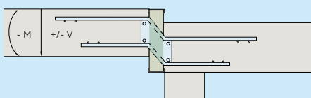
Typenreihe QV Querkraftelemente mit Versatz Seite 33 – 34
