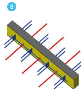
Querkraftanschluss mit Normalkraft z.B. QC- N +240
