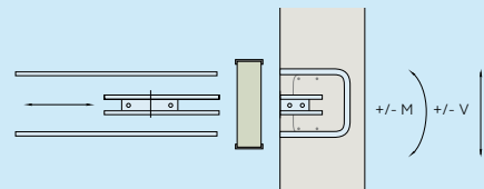
Typenreihe WN / WQ Wandanschlüsse Seite 43 – 44
