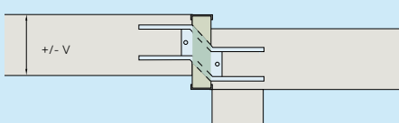
Typenreihe S Erdbebenelemente Seite 46
