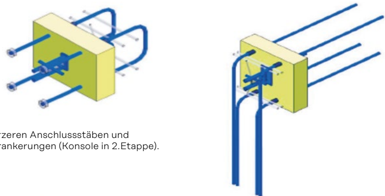
Mit Zugbügelverlängerung in 1. Etappe.
